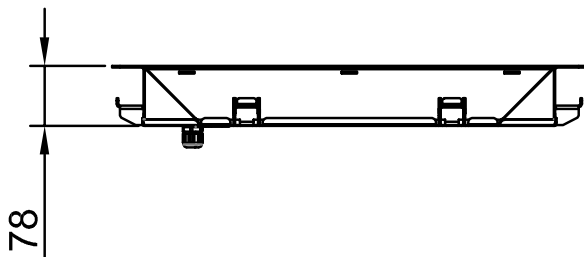
Zij aanzicht
